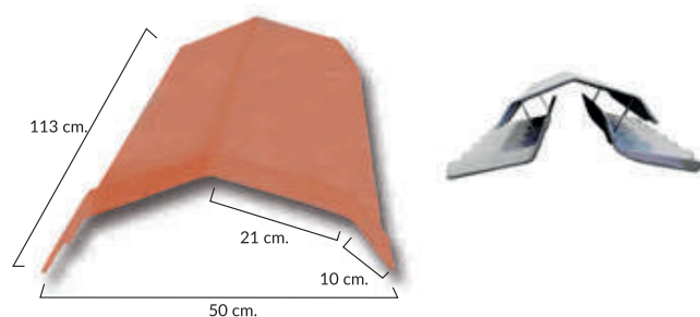
CABALLETE ARTICULADO DIENTE SIERRA
