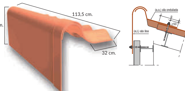
LIMA DE CIERRE
